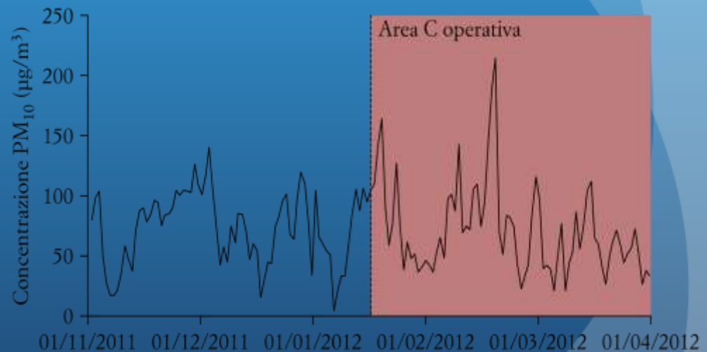
FIG. 5. Andamento della concentrazione media di Pm10 nelle centraline di rilevamento site nel territorio metropolitano di Milano, prima e dopo l'introduzione della cosiddetta «Area C».
